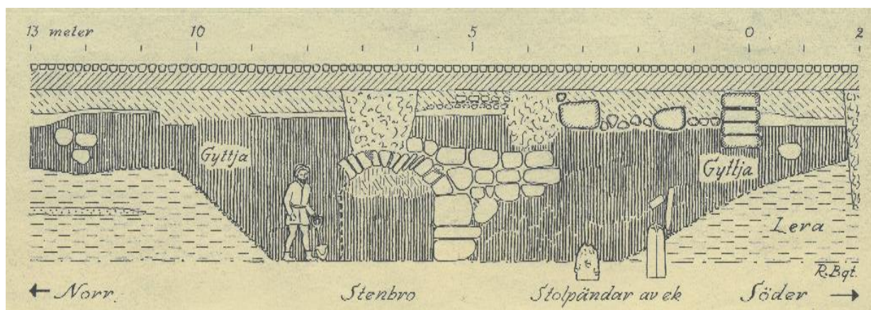
Figur 4. Sektion genom vallgraven med stenbron som lett ut ur staden vid Bredgatan. Uppmätt av Ragnar Blomqvist vid arkeologisk övervakning av kloakgrävning år 1944 (Kulturens LA-arkiv).
