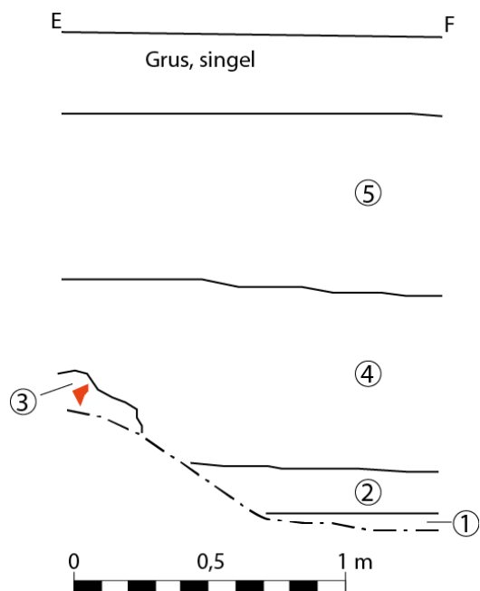
Bilaga 4. Sektion E–F, för referens se bilaga 2.
