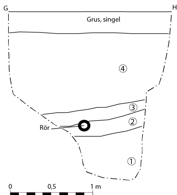
Bilaga 6. Sektion G–H, för referens se bilaga 2.
