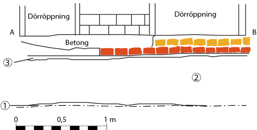
Bilaga 3. Sektion A–B, för referens se bilaga 1.
