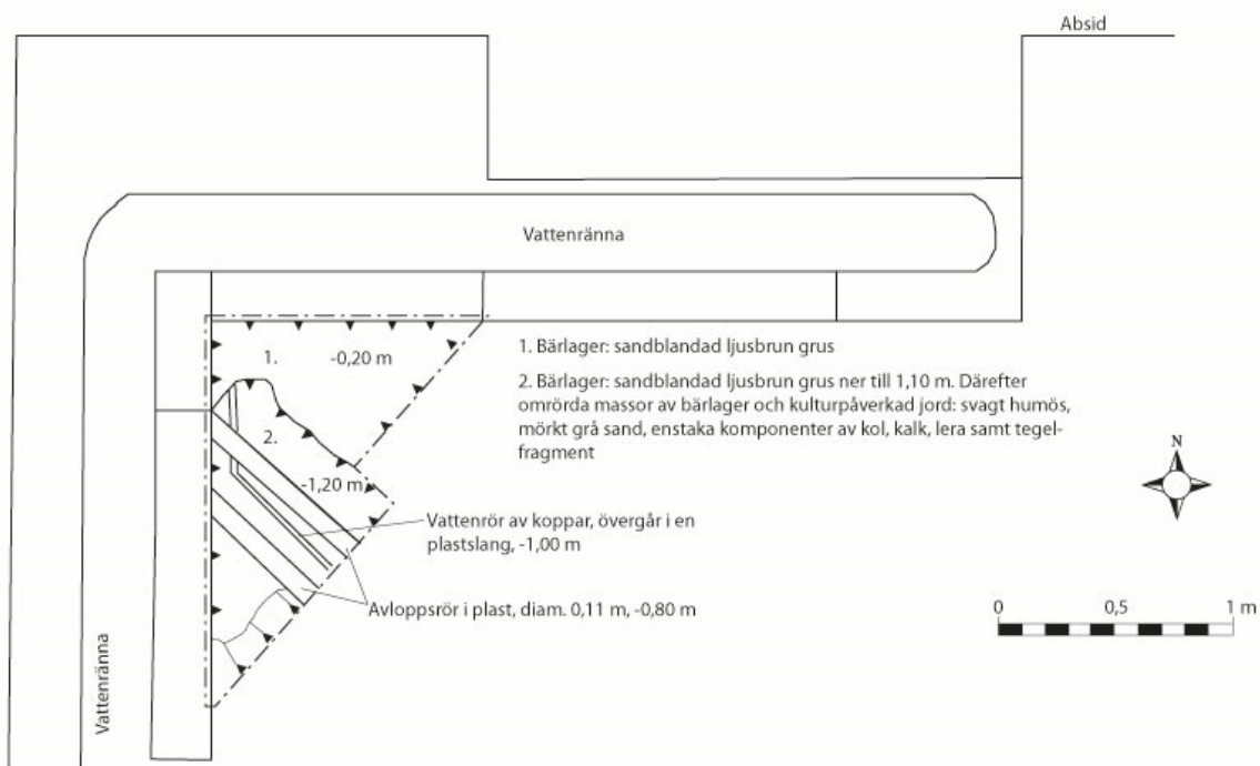
Figur 9. Planritning över schaktningsområdet, med lagerbeskrivning.
