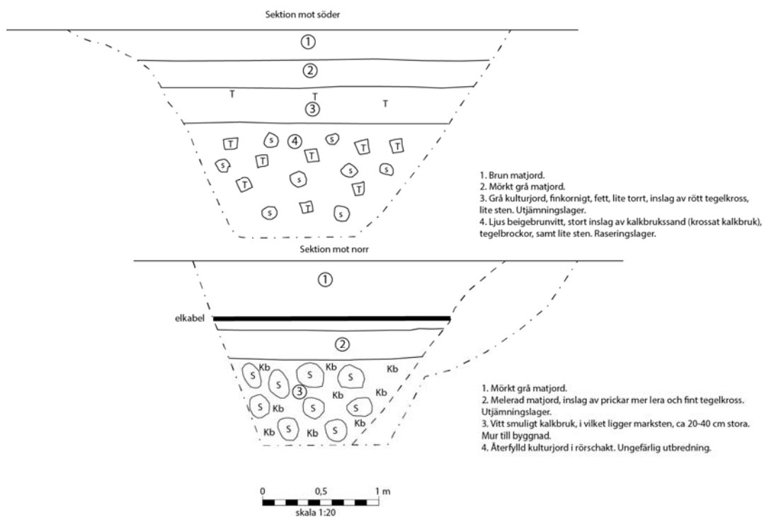
Figur 14. Sektionsritningar med lagerbeskrivning.
