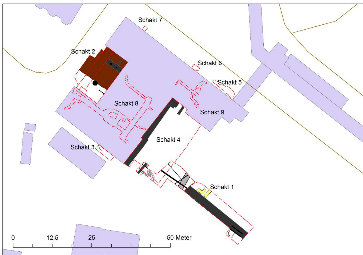
Figur 4. Schaktöversikt.
