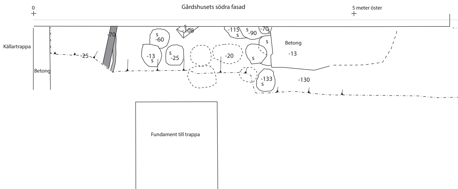
Bilaga 2g. Plan över schakt söder om gårdshuset.
