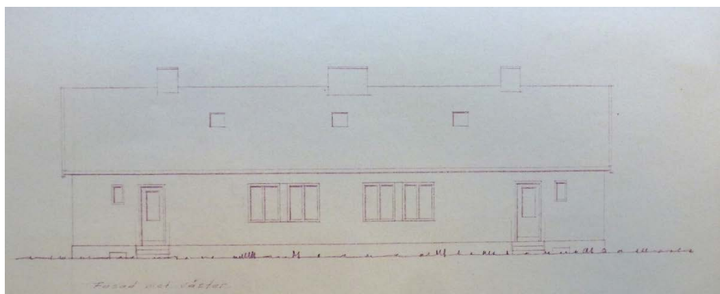
Figur 8. Ritning fasad mot väster vid ombyggnad 1954, upprättad av LBF.
