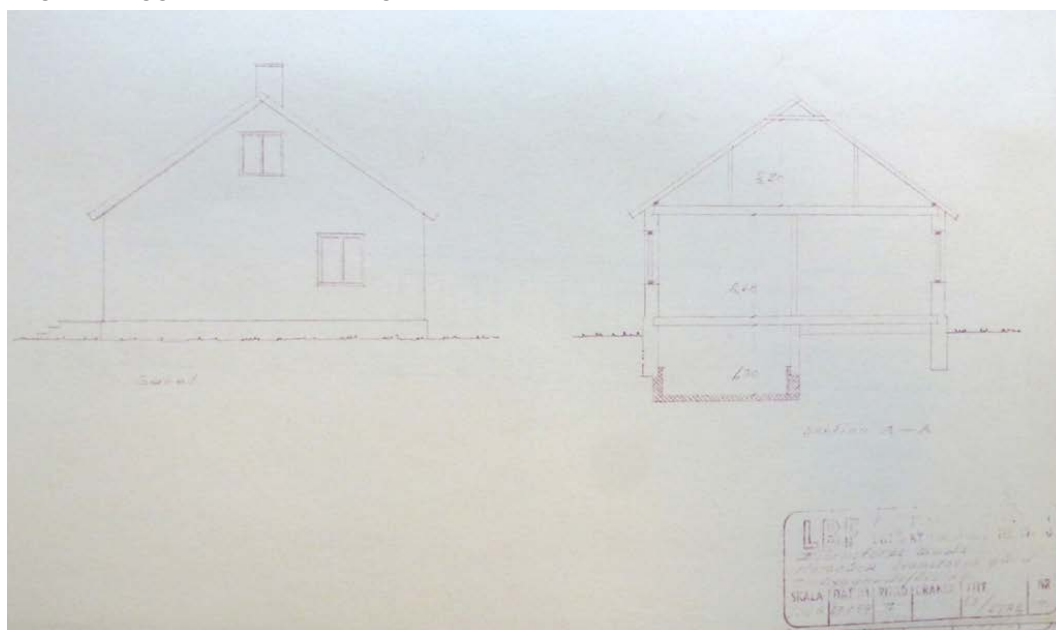
Figur 6. Gavel och sektion 1954 upprättad av LBF. Mått vindsplan 2,30, bottenplan 2,68, källarplan 1,90.
