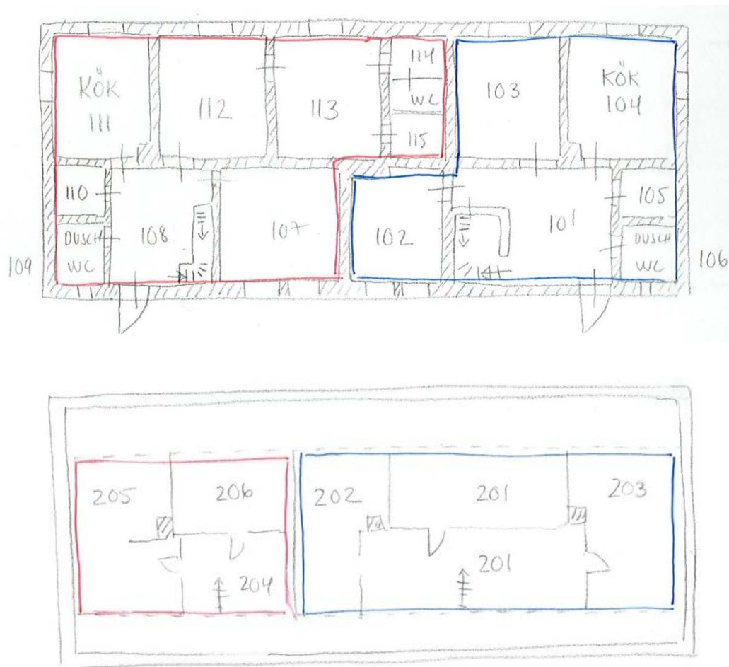
Figur 10. Skiss över dagens (2014) planlösning bottenvåningen och vindsvåningen. Ej skalenlig. Västra lägenheten markerad med rött och östra med blått. Skiss utförd av Carita Melchert.
