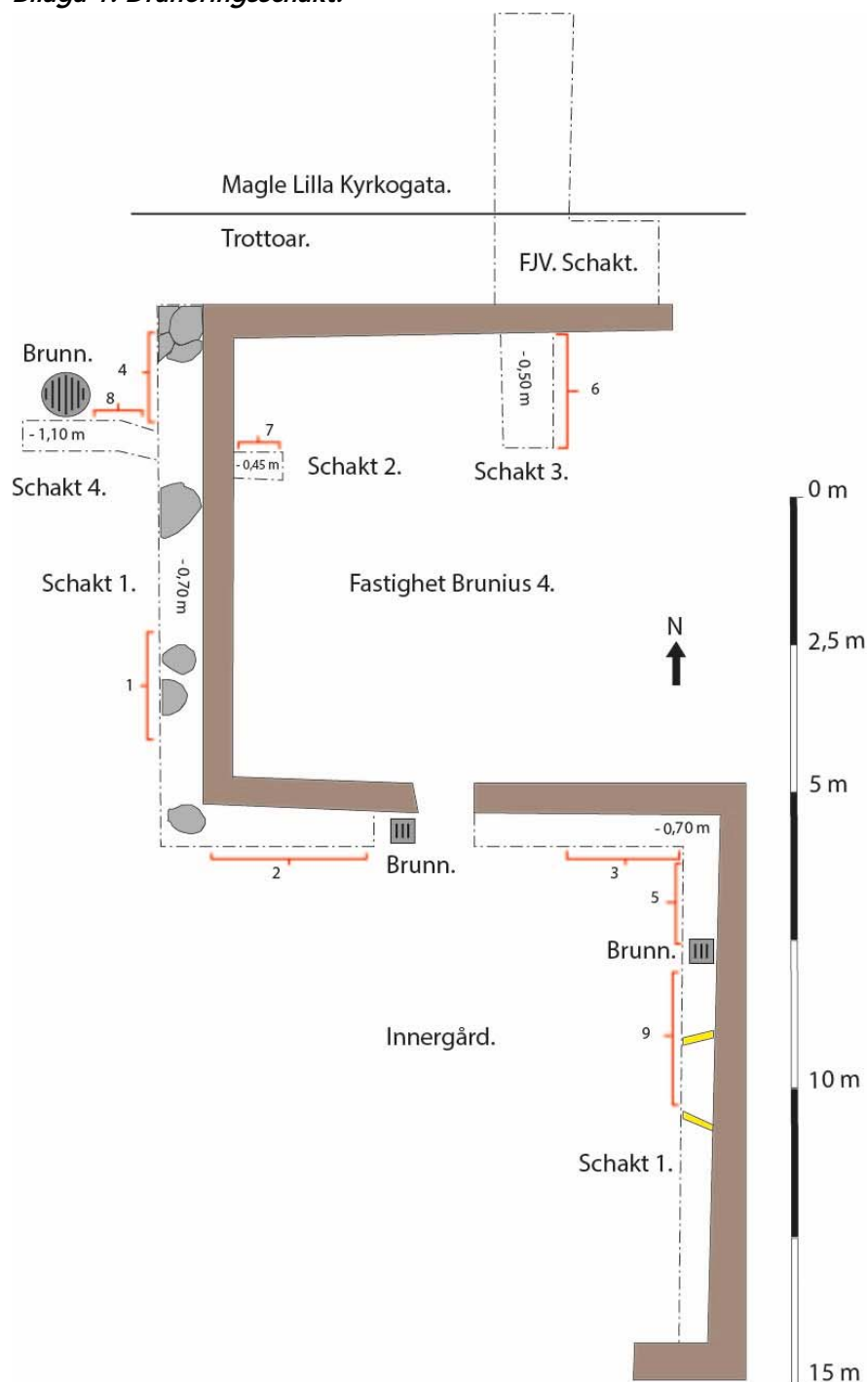
Bilaga 1 Planritning över dräneringsschakten fas 1. Sektionerna är markerade med orangea sträck. Ledningar är markerade med gult.
