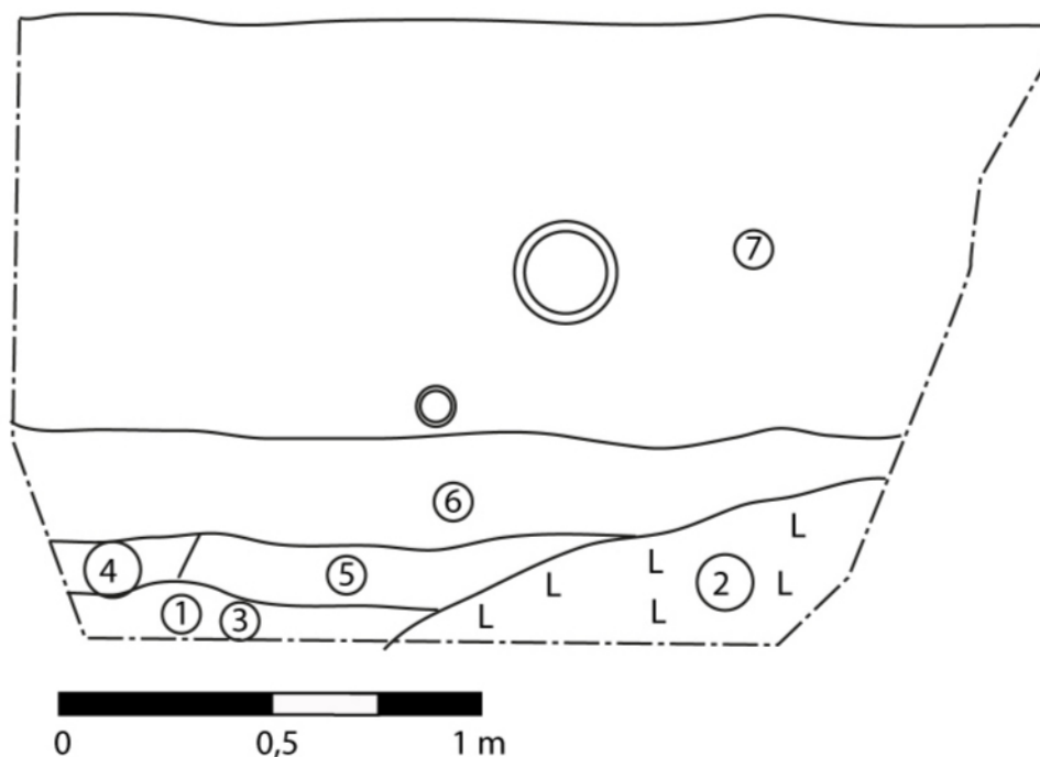
Sektionsritning över den västra schaktkanten av schaktet för fettavskiljaren
