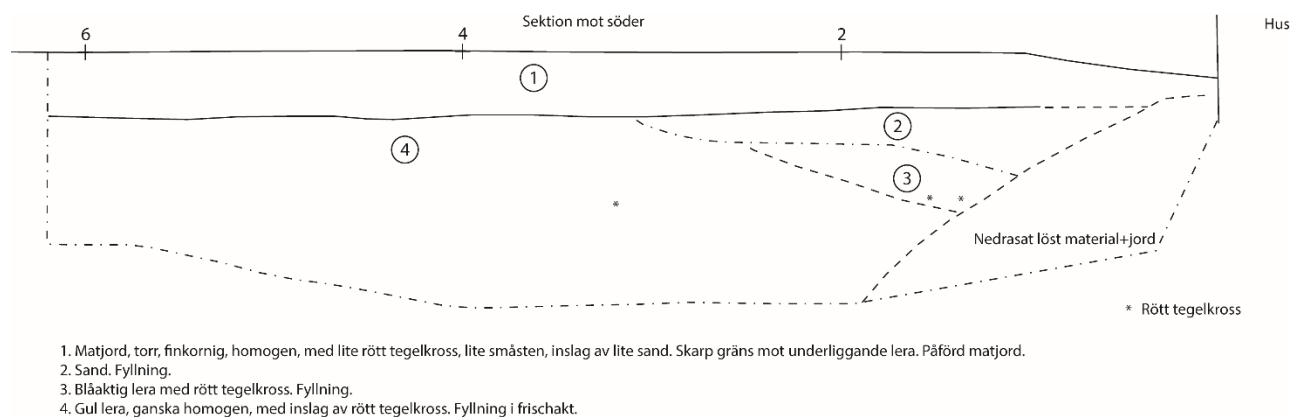
Figur 6. Sektion mot söder, ca 2,3 m från gårdshusets östra fasad.
