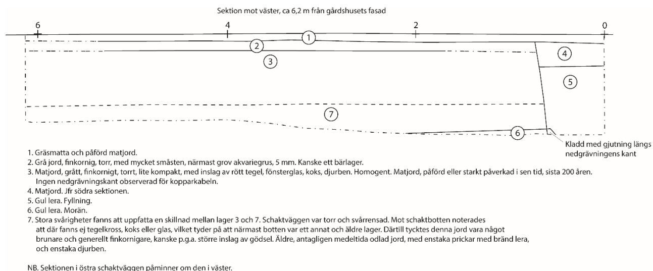
Figur 4. Sektion mot väster, ca 6,2 m från gårdshusets östra fasad.
