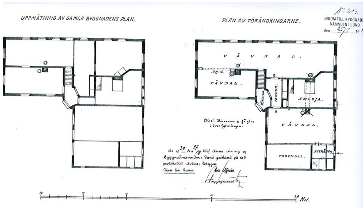
Bottenplan 1930. Källa: Arkiv Kulturen i Lund.
